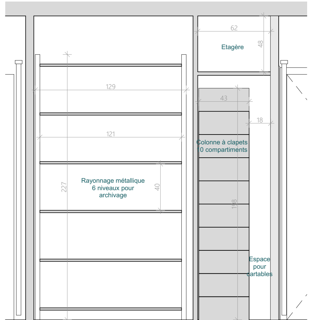
Proposition 3 - Coupe A4 - 20ème
