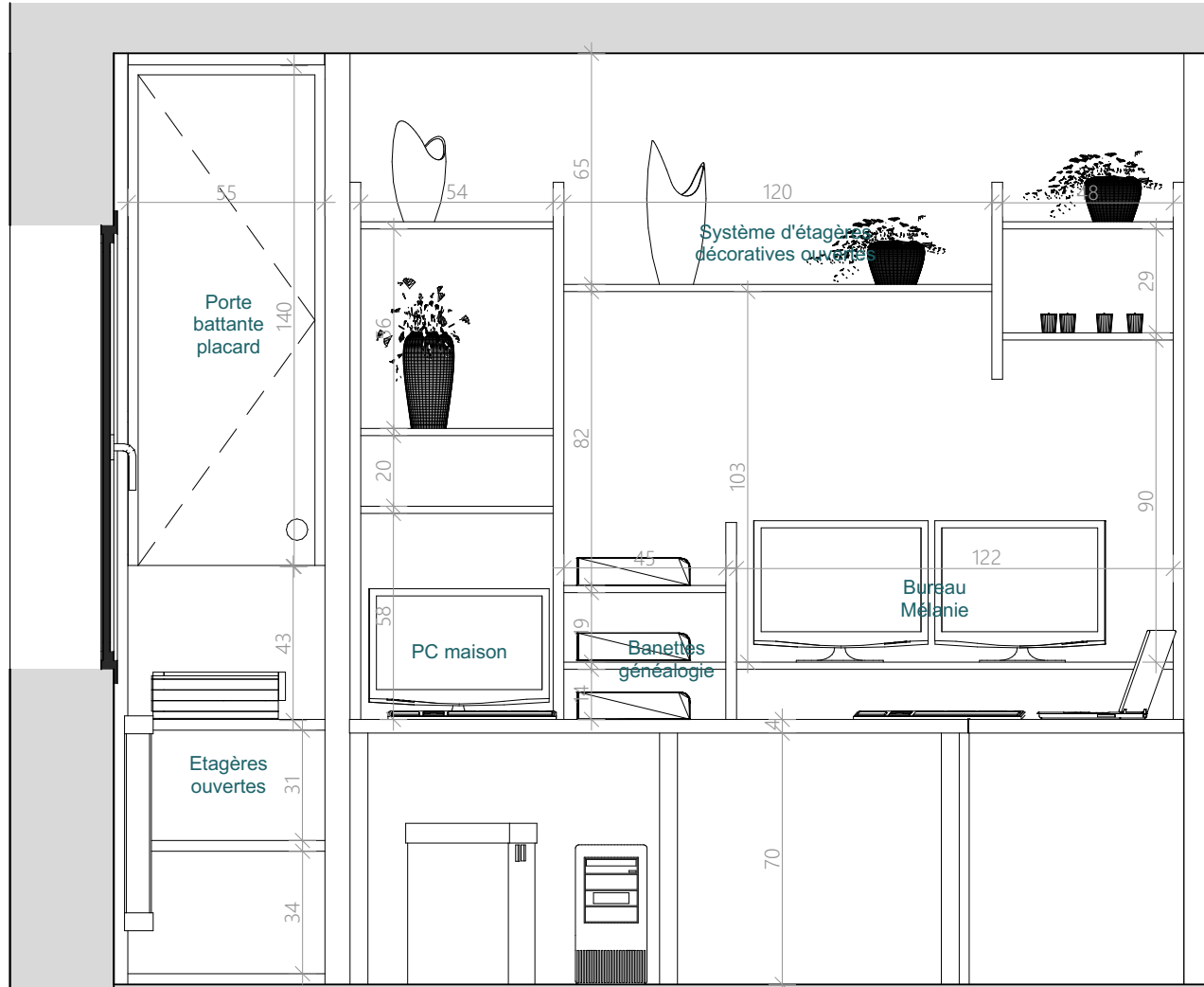
Coupe A1 - Propo 1 - 20ème
