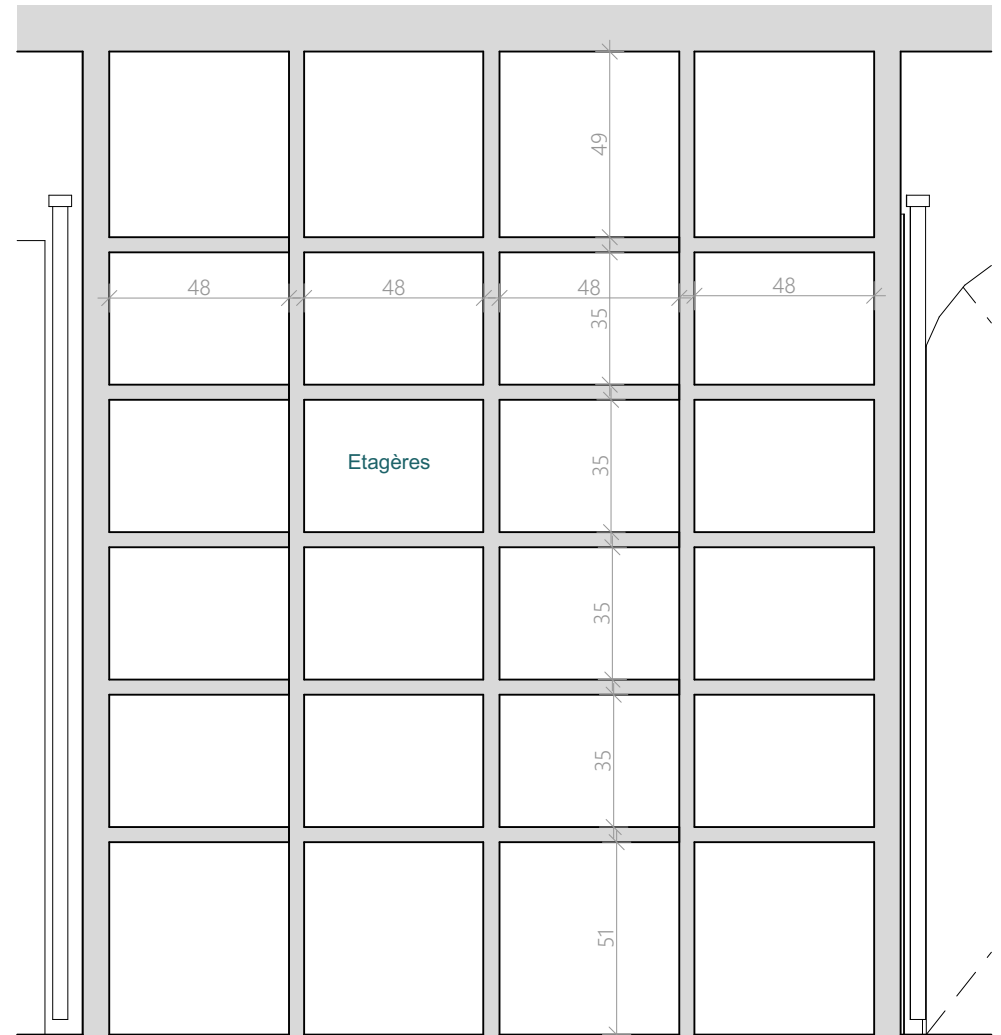
Proposition 2 - Coupe A4 - 20ème
