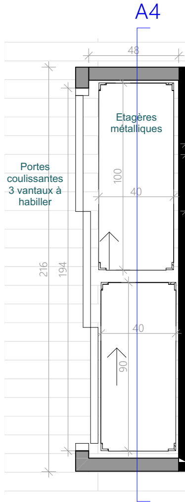
Proposition 1 - Plan - 20ème
