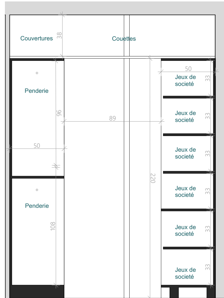
Proposition 3 - Coupe C - 20ème
