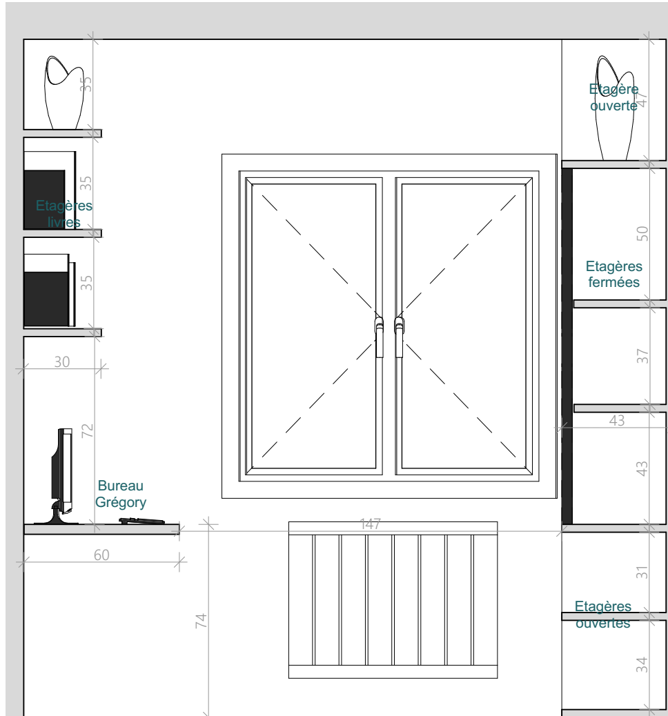
Coupe C2 - Propo 2 - 20ème
