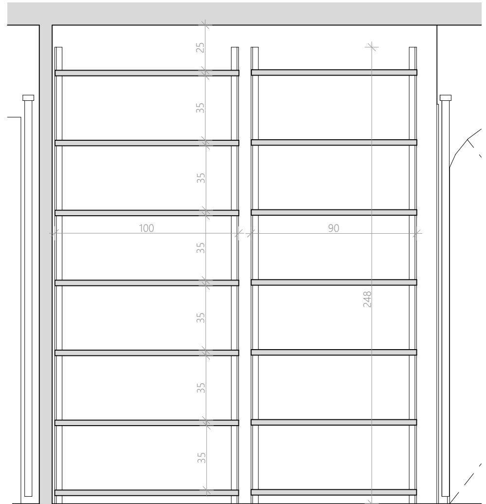
Proposition 1 - Coupe A4 - 20ème
