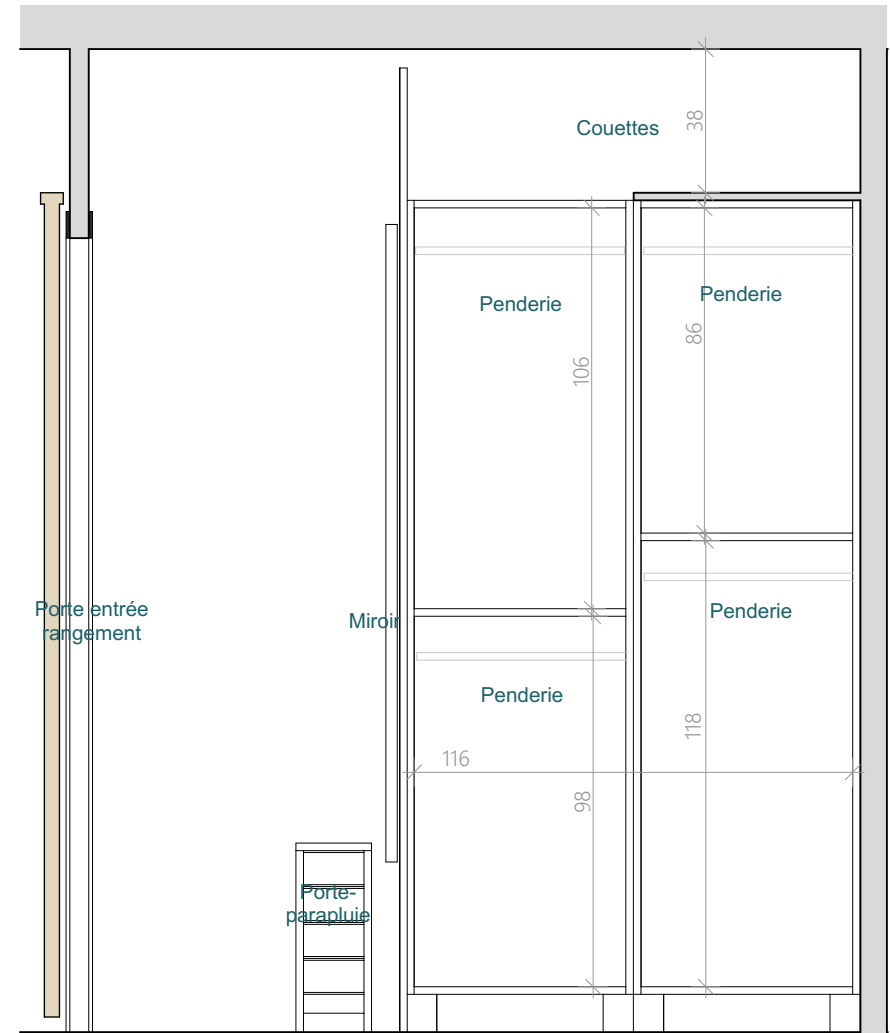
Proposition 3 - Coupe A3 - 20ème
