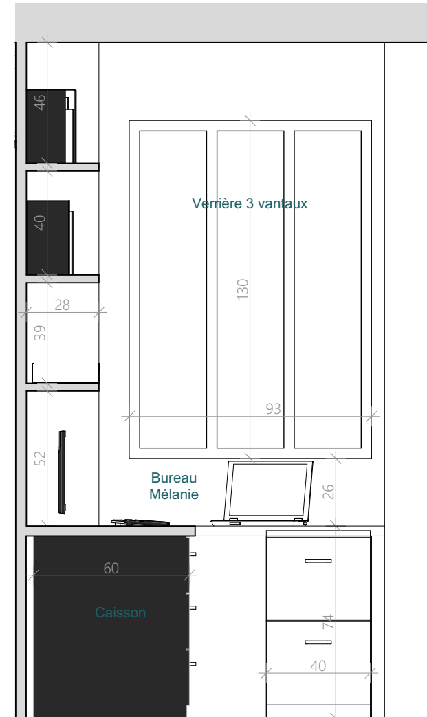
Coupe C1 - Propo 2 - 20ème
