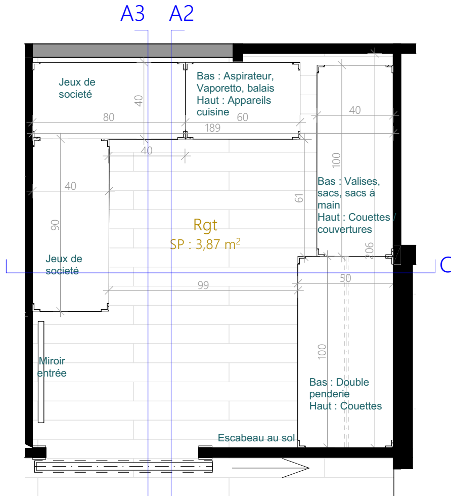
Proposition 1 - Plan - 20ème
