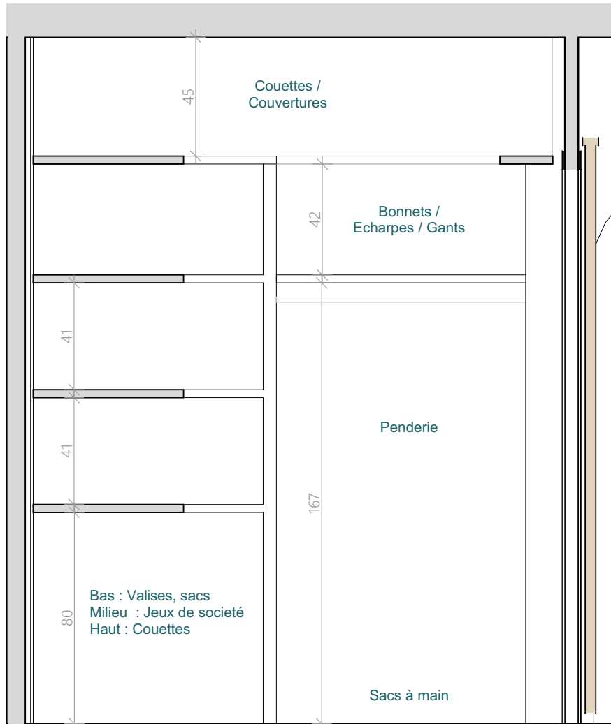
Proposition 2 - Coupe A2 - 20ème
