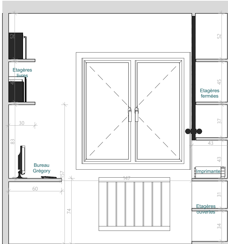
Coupe C2 - Propo 1 - 20ème
