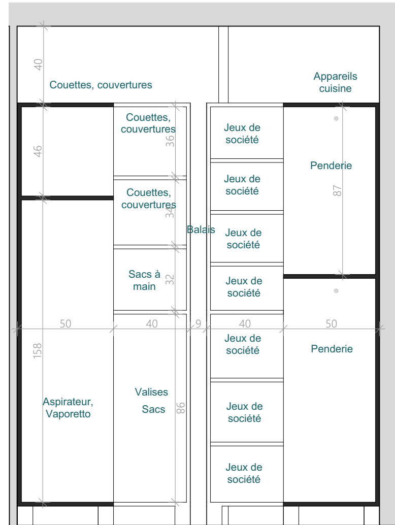
Proposition 4 - Coupe C - 20ème
