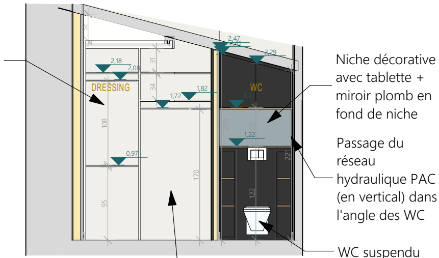
Coupe CC
