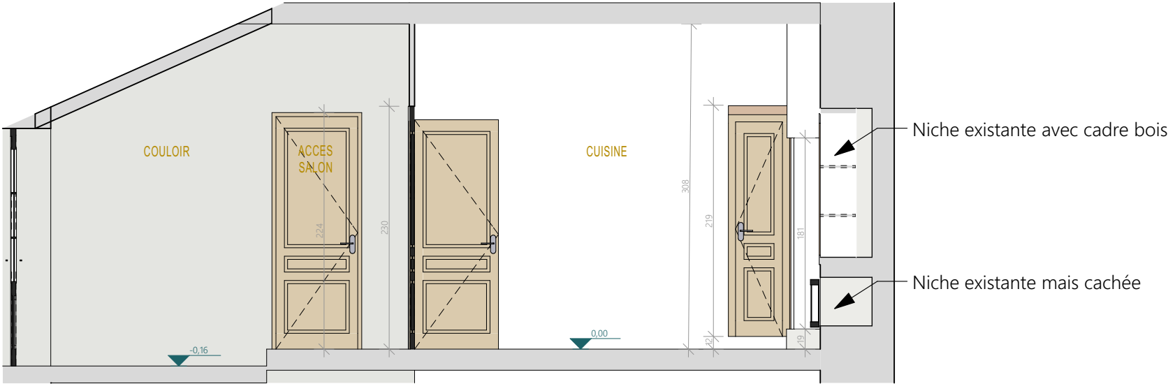
Coupe FF
