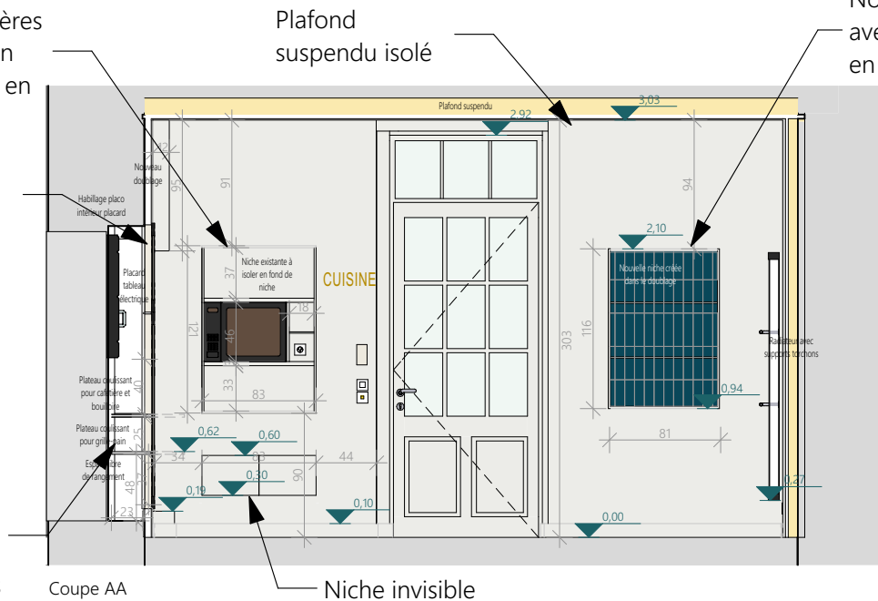
Coupe AA
