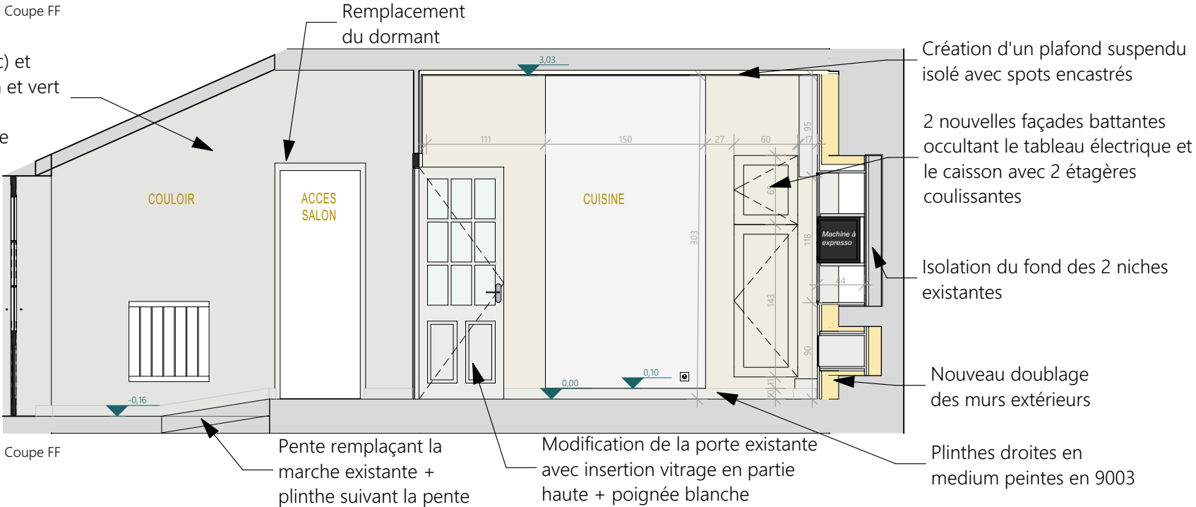
Coupe FF
