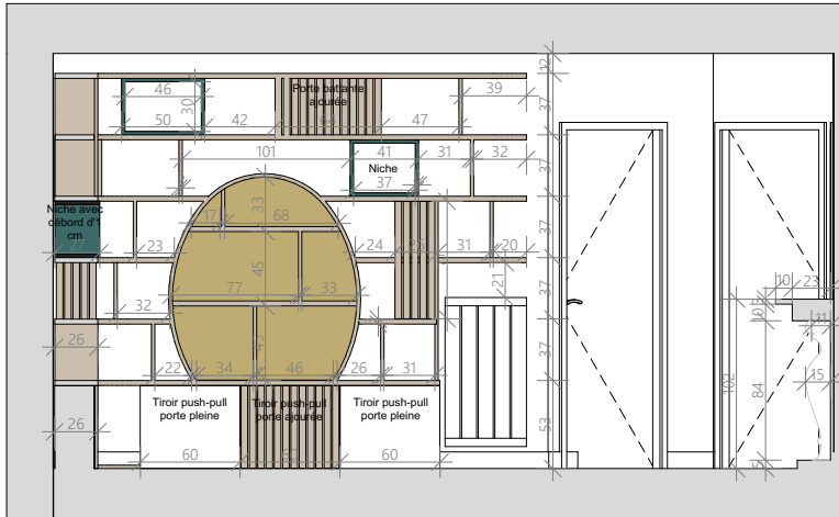
Coupe D
